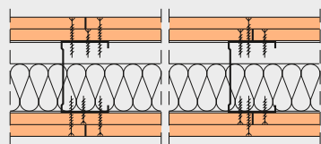
fermacell constructie 1 S 31 – 60 dB met slechts 120 mm wanddikte
